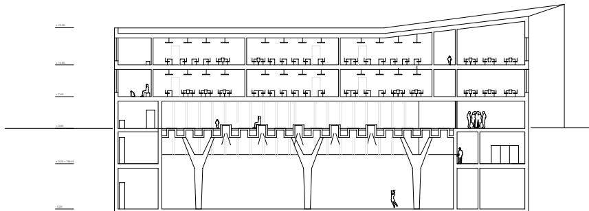
Coupe AA 1:200
